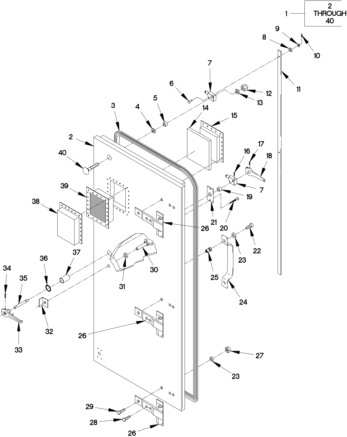
FIGURE 222. VAN RIGHT HAND DOOR
